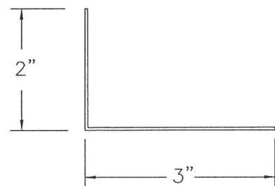
RAKE ANGLE (16 GA. GALV.)
