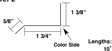
Rake Trim MDLRT
