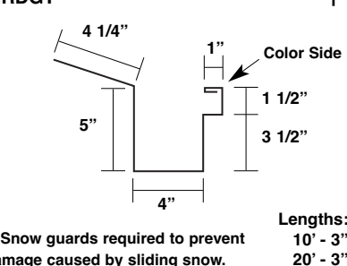
Gutter* MRDGT
