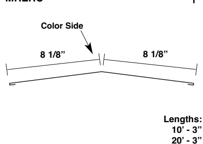
Ridge Trim* MRERC
