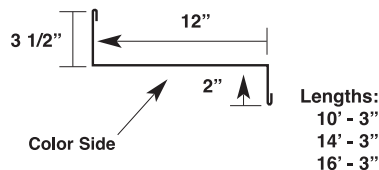
Valley Trim* (P-VF)
