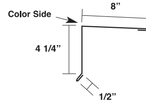
Hi-Side Trim* (R-HS)
