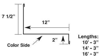
Gutter Apron* (P-GA)
