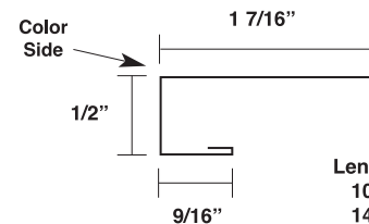
Matrix Soffit J MTSJ
