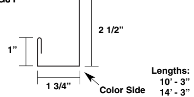
Rake Tie-In Trim MGEW
