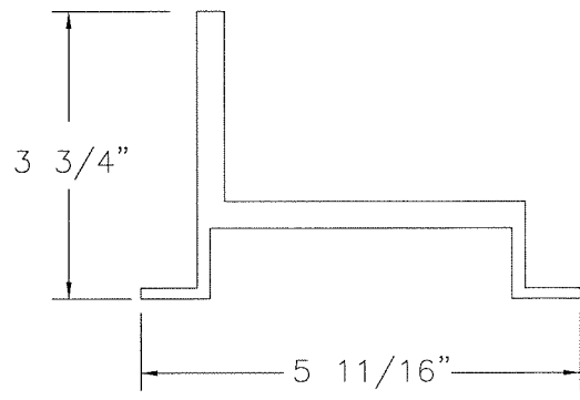
RAKE ANGLE CLIP (16 GA. GALV.)
