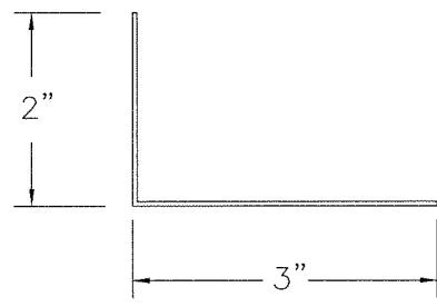
RAKE ANGLE (16 GA. GALV.)
