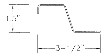
EAVE PLATE (18 GA. GALV.)
