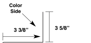
Rake Tie-In Trim MDEW
