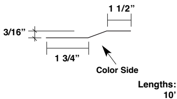
Rake Tie-In Trim MDEW
