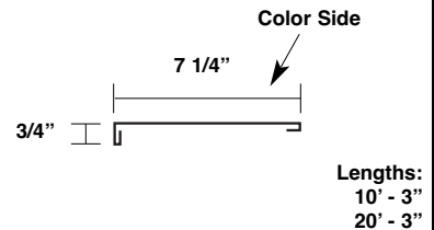
Rake End MLRE
