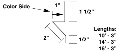
Zee Flashing (P-ZF)
