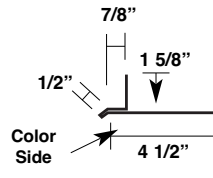
Overhead Door Drip 8" (P-ODP-8)
