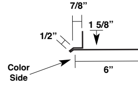
Overhead Door Drip 8 7/8" (P-ODP-8 7/8)
