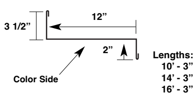
Valley Trim* (P-VF)
